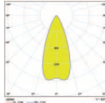
CURVA POLAR 25°
