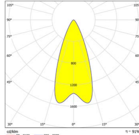
CURVA POLAR 25°
