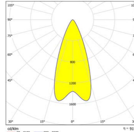
CURVA POLAR 25°
