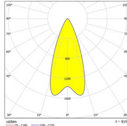
CURVA POLAR 30°
